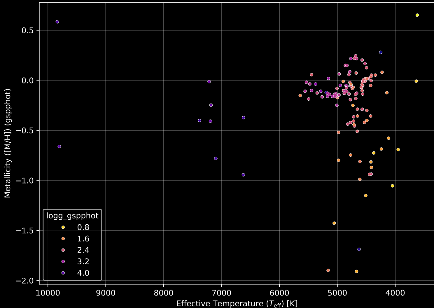
APOGEE DR17 Field: [340-14] Stellar Population Parameters (n= 127)
